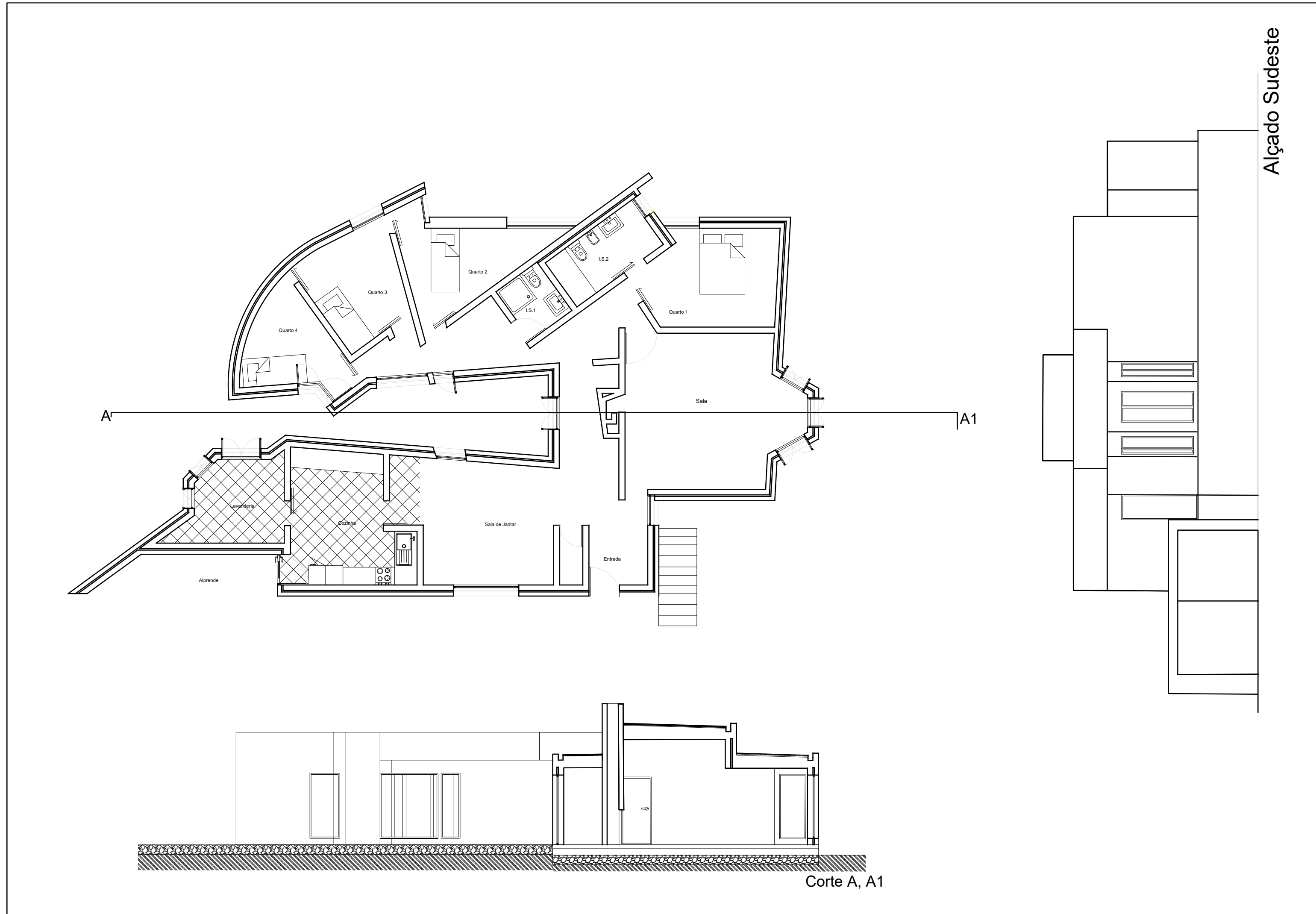
PLANTA À ESCALA 1:100
