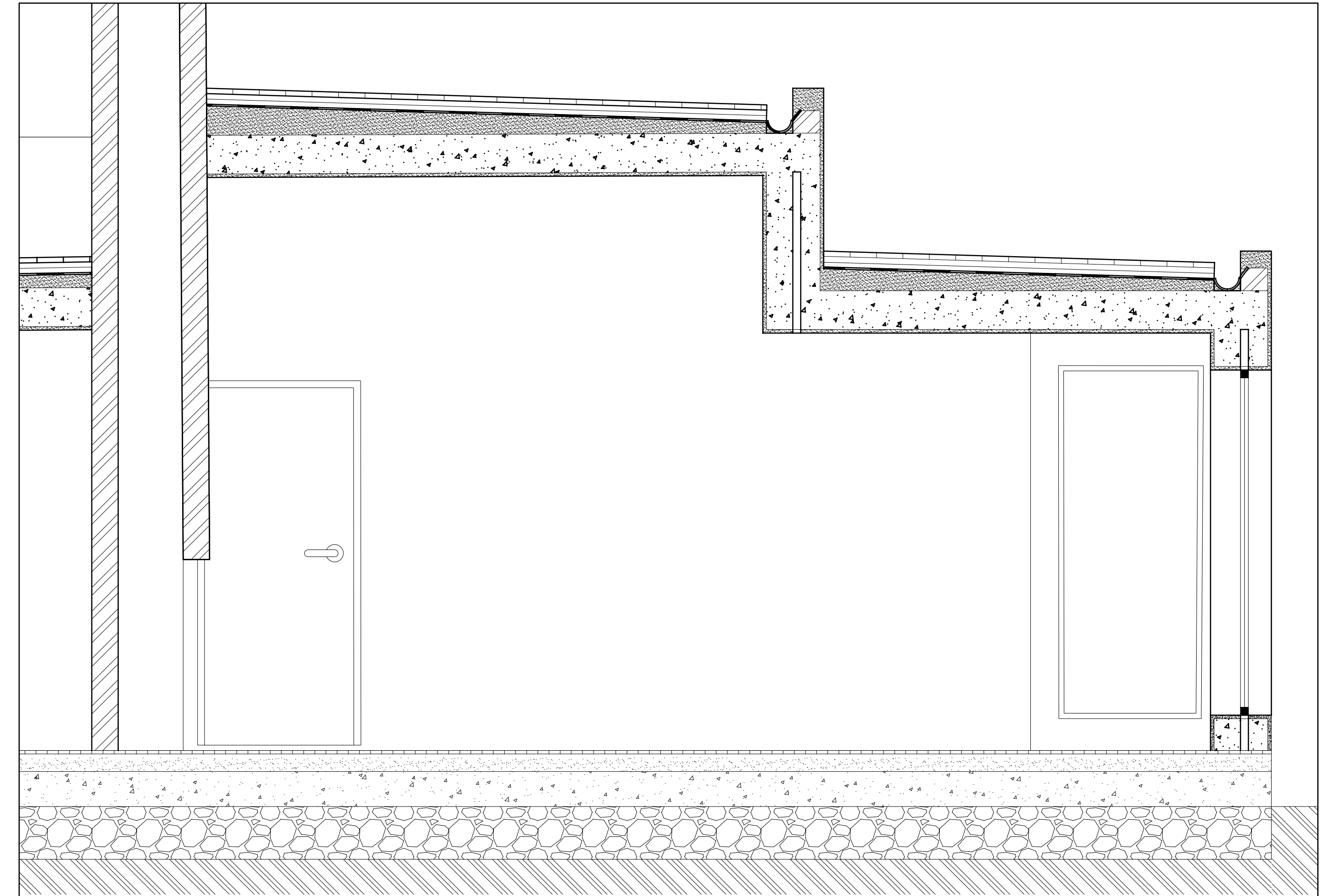
CORTE A, A1 À ESCALA 1:20
