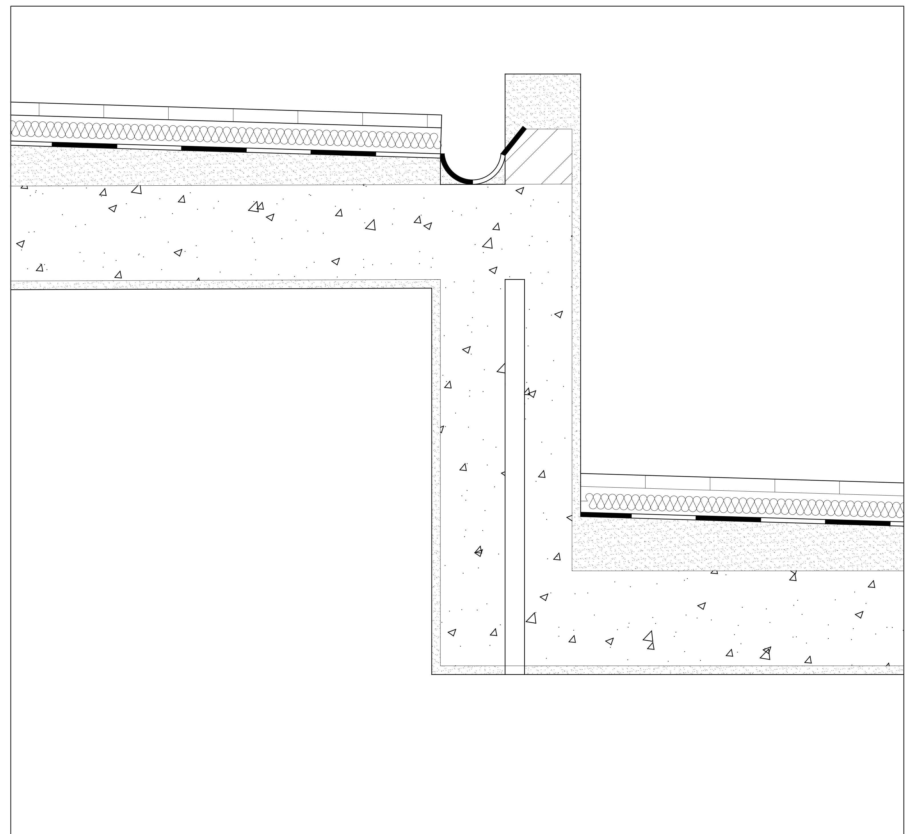
PORMENOR DO TELHADO 1:5
